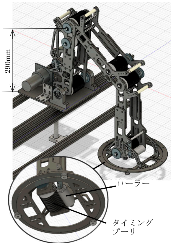
図3 除草部
